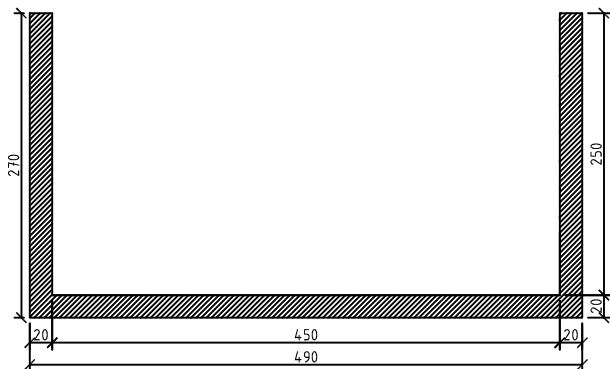
SECTIUNE A-A
