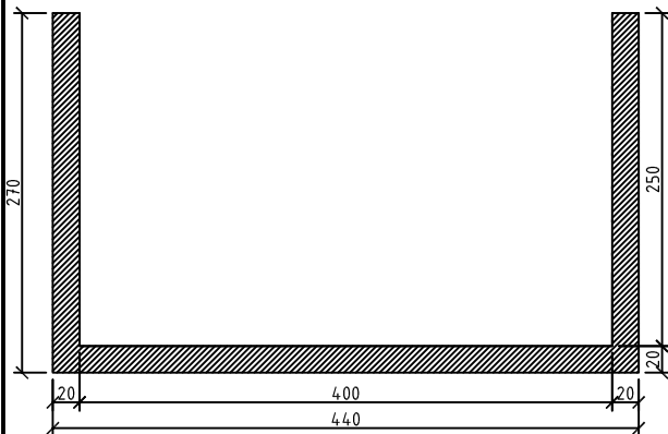
SECTIUNE A-A
