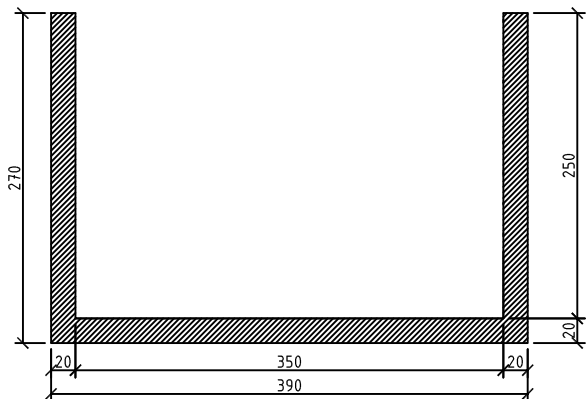
SECTIUNE A-A
