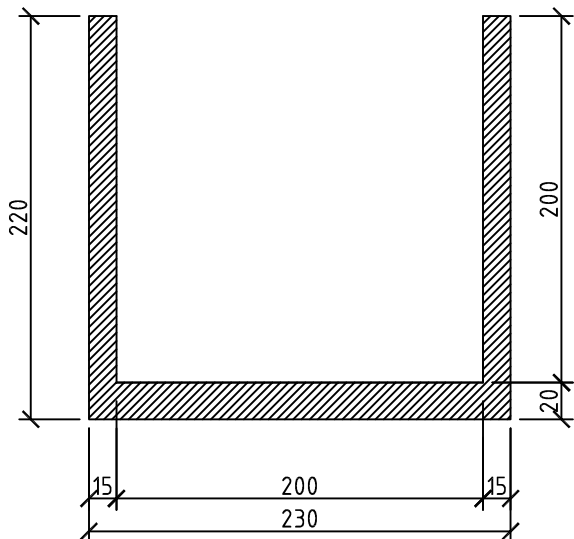
SECTIUNE A-A
